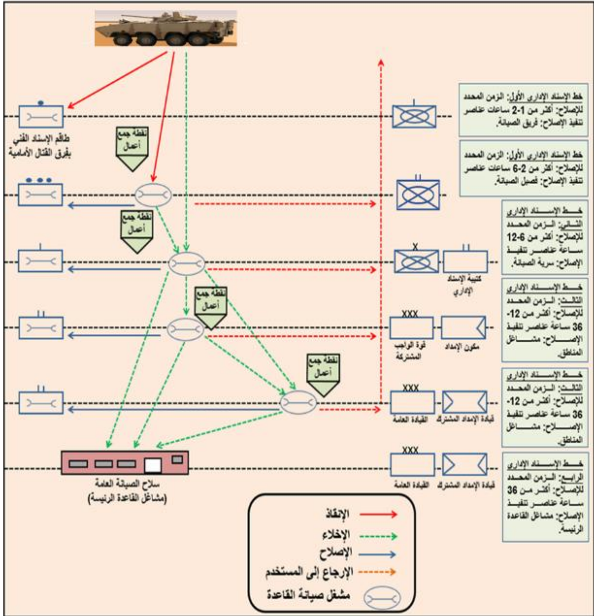
الشكل رقم (39) مخطط الإنقاذ والإصلاح والإخلاء
